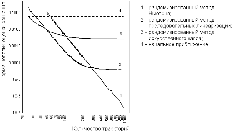
Рис 1. Зависимость нормы невязки от числа траекторий на одном из примеров
